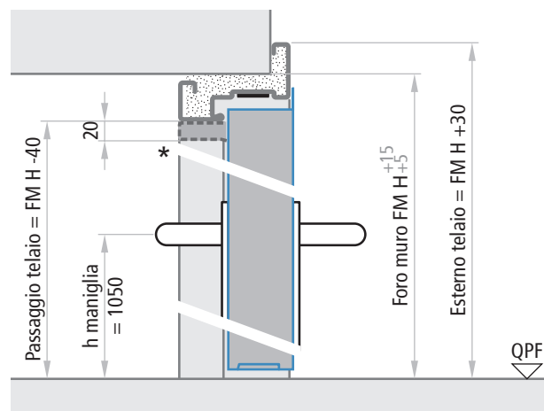
Porta senza battuta inferiore Sezione verticale
