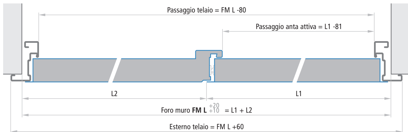
Porta a due ante Sezione orizzontale
