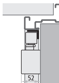
RC2-G PROGET (lato a spingere)
