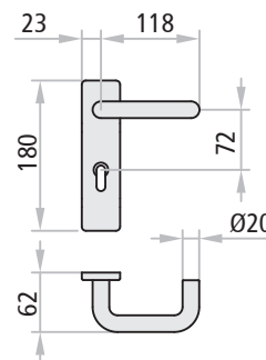
Maniglia M1R in plastica nera
