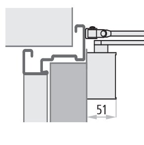
CP1 PROGET (lato a tirare)
