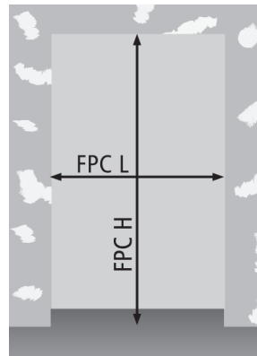
Foro Parete cartongesso
