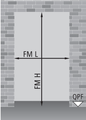
Porta ad un'anta FM L x FM H
