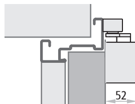
CP2 PROGET (lato a tirare)
