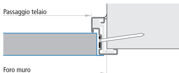
Porte EI 2 60, REI 60 e REI 120
