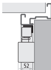
RC2-G PROGET (lato a spingere)
