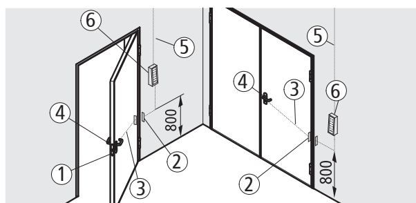
Schema componenti
