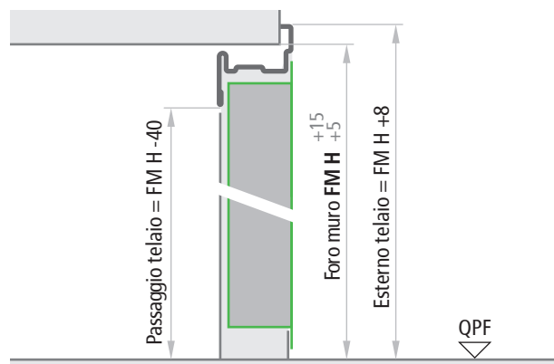
Porta senza battuta inferiore Sezione verticale
