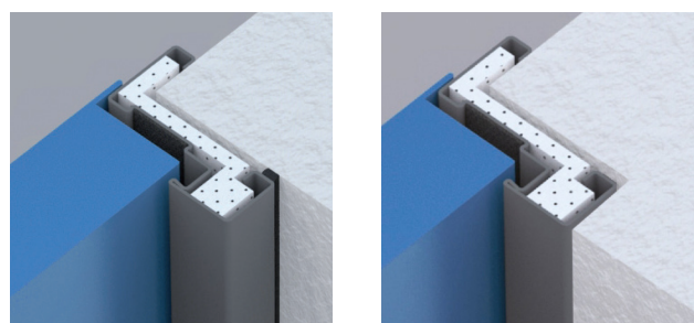
Porte EI 2 60, REI 60 e REI 120
