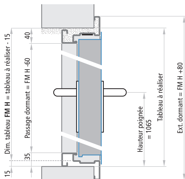
Coupe verticale
