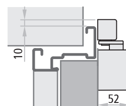
RC2 PROGET (côté tirant)
