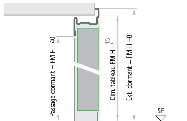
Porte sans battue inférieure - Coupe verticale
