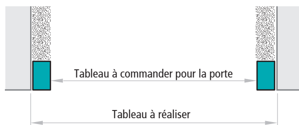
Coupe horizontale
