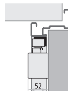
CP2-G PROGET (côté poussant)
