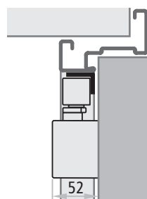
RC2-G PROGET (côté poussant)
