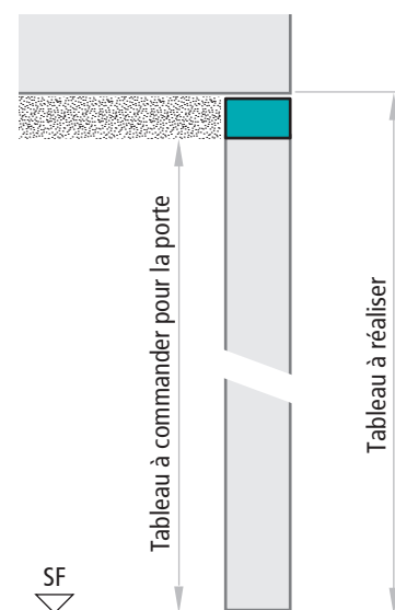
Coupe verticale
