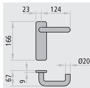
version pour porte Univer/Proget
