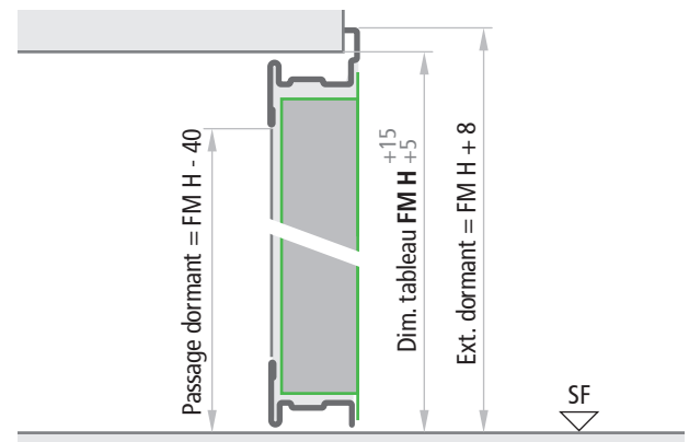
Porte avec battue inférieure interne Coupe verticale
