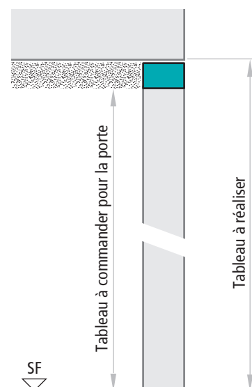
Coupe verticale
