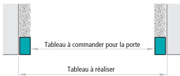
Coupe horizontale
