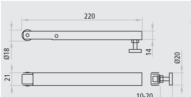
Bras accompagnateur pour vantail passif
