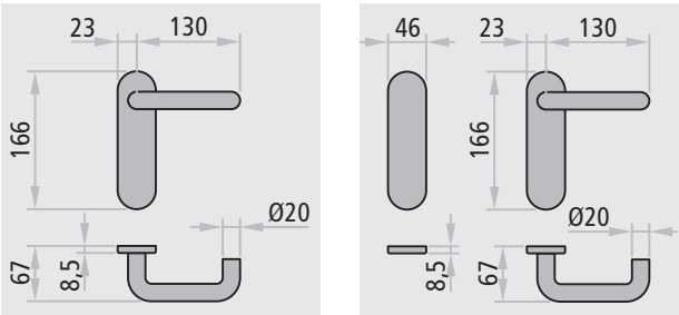
version pour porte Univer/Proget version pour porte Rever
