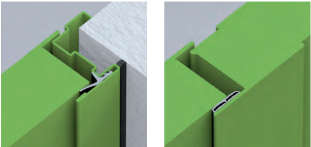
Dormant périmétral
