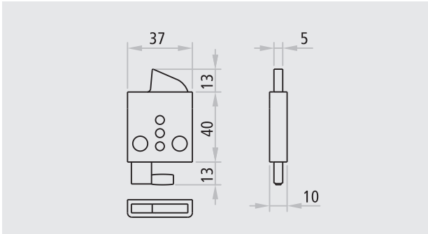
Dispositif haut pour vantail passif UNIVER et REVER
