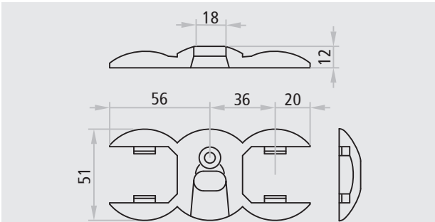
Gâche de sol vantail passif REVER
