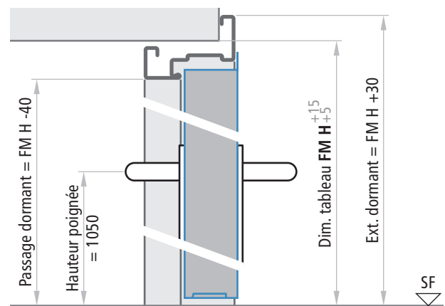
Porte sans traverse inférieure - Coupe verticale
