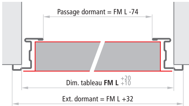
Porte à un vantail - Coupe horizontale
