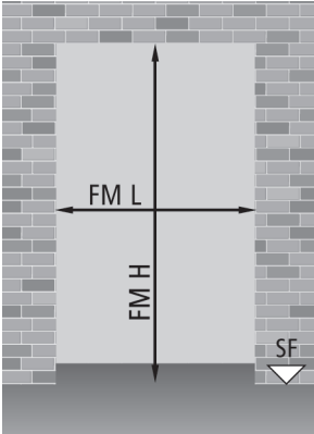
Porte à un vantail FM L x FM H
